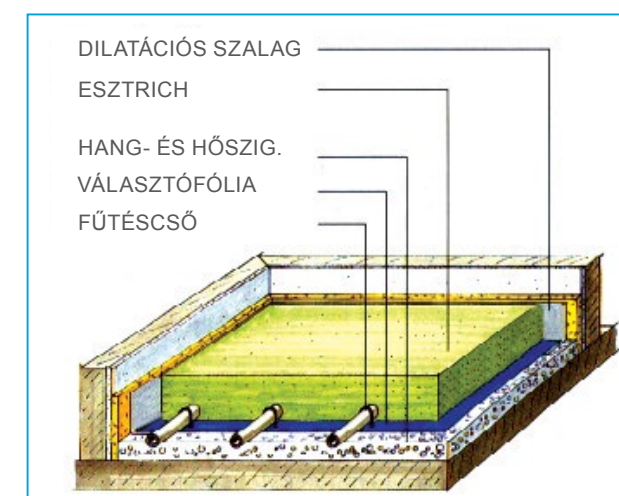
hűtött/fűtött esztrich
