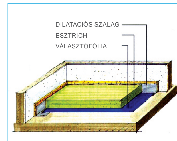
csúsztatott esztrich
